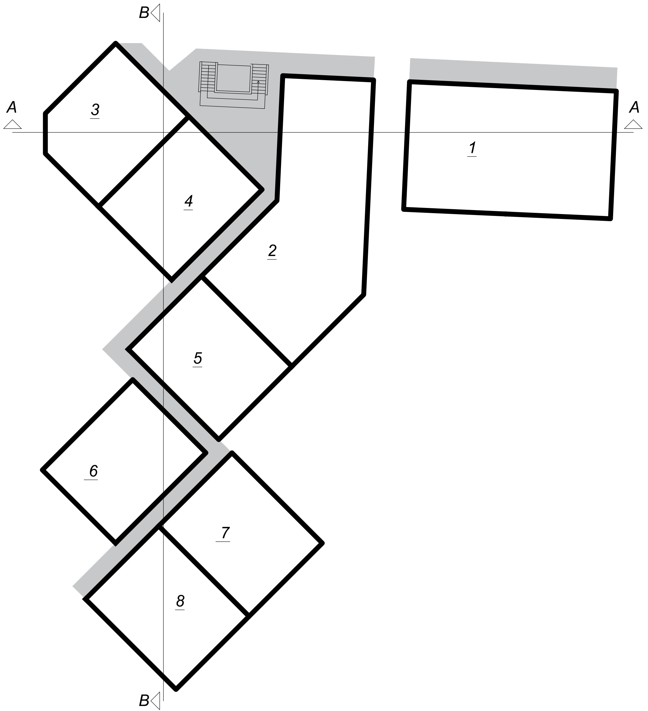
Beganegrondvloer App.1- 8 (1:200)
