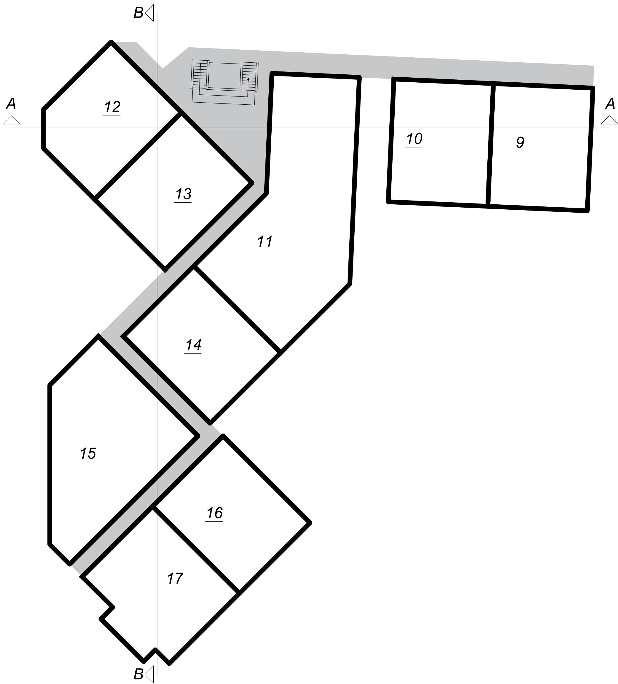
1 verdiepingsvloer App.9- 17 (1:200)
